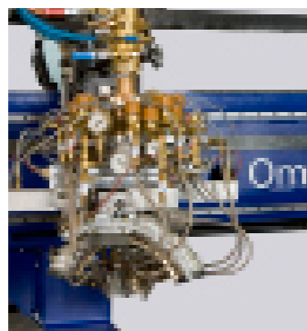
Oxicorte com chanfrador multimaçaricos DAFL. Ângulos ajustados via CNC de 15° a 60°. Giro infinito para chanfros com espessura de até 80 mm.
